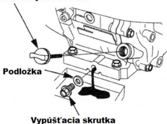
Zátka oleja s mierkou
